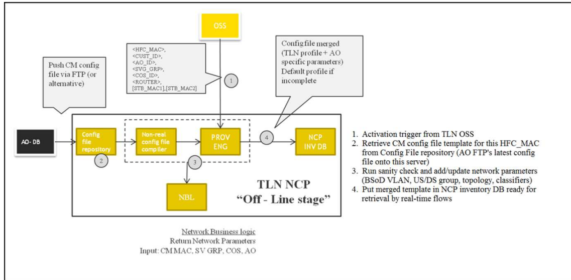
Figure 7-1: AO Docsis CPE modem configuration
